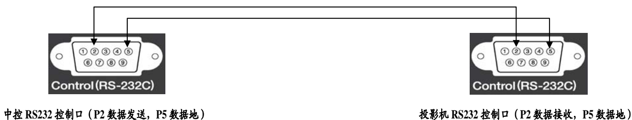
EPSON投影机RS232 控制连接图
